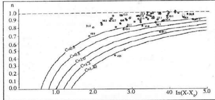
Figure 3 : Graphe de la relation n = f[\ln(X - X_0)] de la r. Aché - s. Aché, F = 282 \text{ km}^2 , N = 62 crues.
